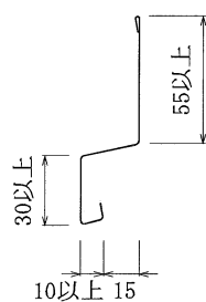
断面詳細図
